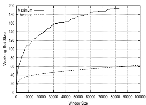
(c) SPARC, GCC, 276 pages.
