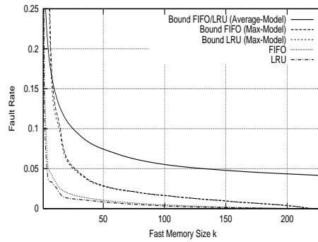
(d) SPARC, COMPRESS, FIFO and LRU.
