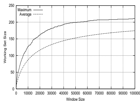
(d) SPARC, COMPRESS, 229 pages.
