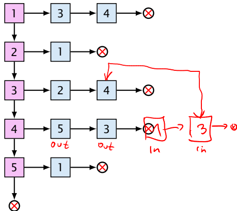
Adjazenzliste
