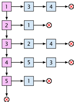
Adjazenzliste
